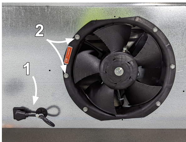
Fig. 29 Fan basket
