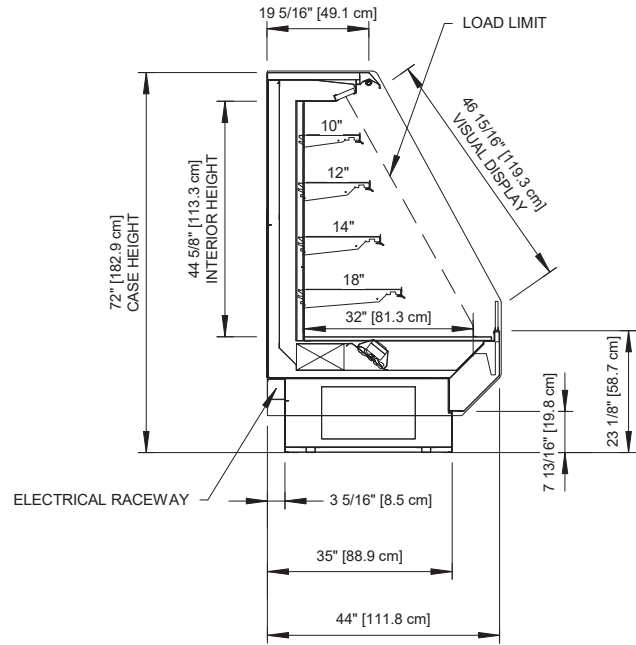
7 13/16" TOEKICK (OPTIONAL)
