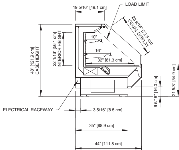
6 15/16" TOEKICK
