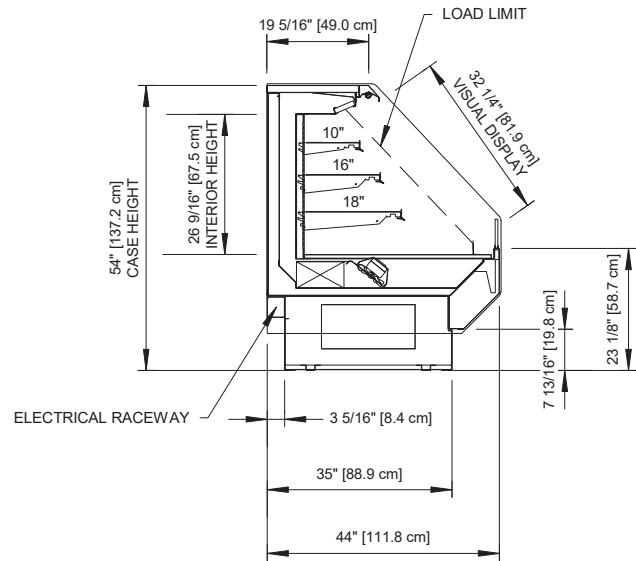
7 13/16" TOEKICK (OPTIONAL)
