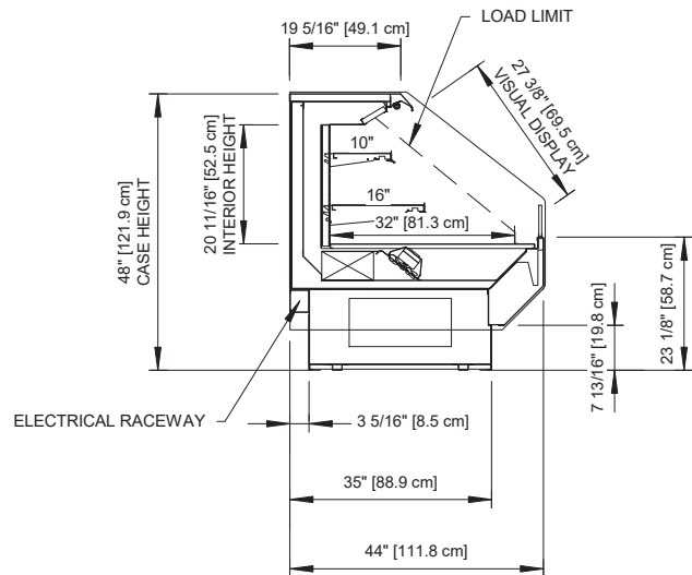
7 13/16" TOEKICK (OPTIONAL)
