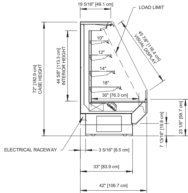
7 13/16" TOEKICK (OPTIONAL)
