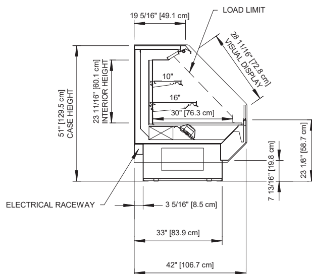
7 13/16" TOEKICK (OPTIONAL)
