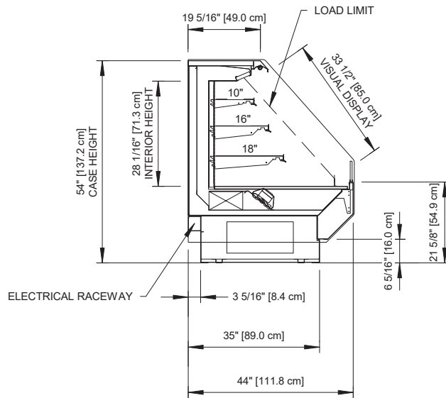
6 5/16" TOEKICK
