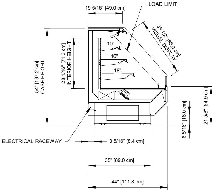
6 5/16" TOEKICK
