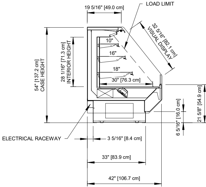
6 5/16" TOEKICK
