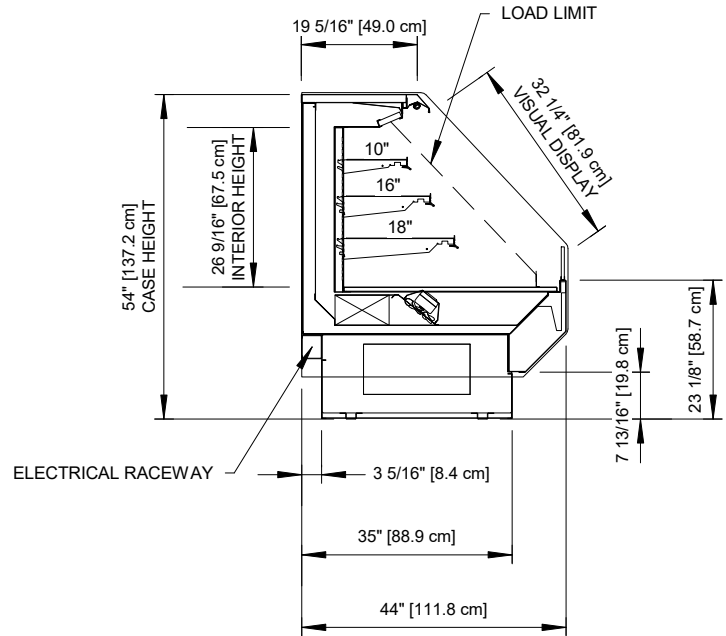
7 13/16" TOEKICK (OPTIONAL)
