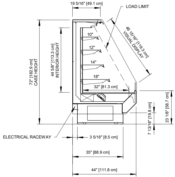
7 13/16" TOEKICK (OPTIONAL)
