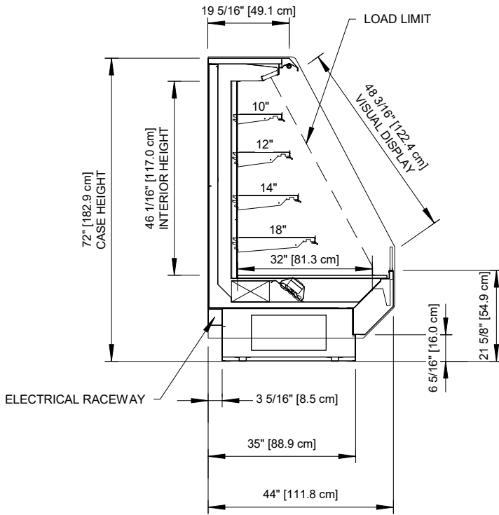
6 15/16" TOEKICK
